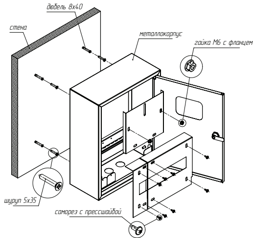
Рис. 1 - Схема монтажа
