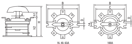
Рис. 7 Пакетные переключатели серии ПП – Исполнение 1
