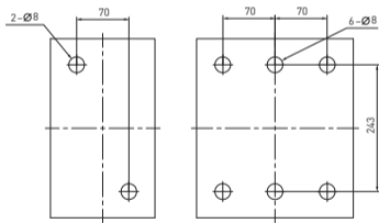
Габаритные размеры ВА-99М 1250 с электронным распределителем
