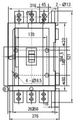
Габаритные и установочные размеры ВА-99М 1250А
