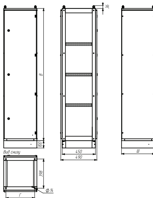
Рис.1 - Общий вид шкафов ВРУ-1 Unit S
