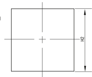
Установочные размеры (отверстие в панели щита)
