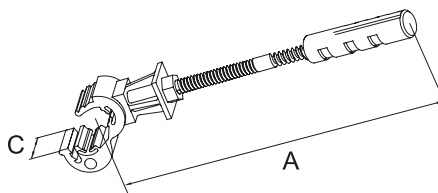
Держатель фасадный пластиковый с дюбелем
